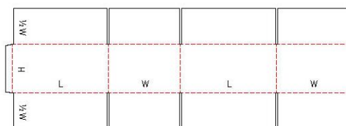
Lepený nebo šitý spoj
